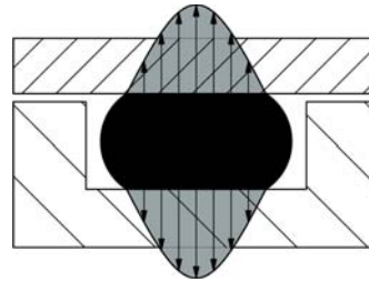
O-Ring unter Druck
