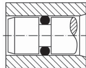
radial verpresst, außendichtend
